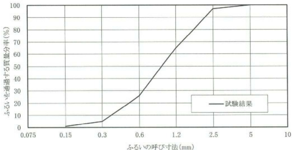
粒度分布曲線
